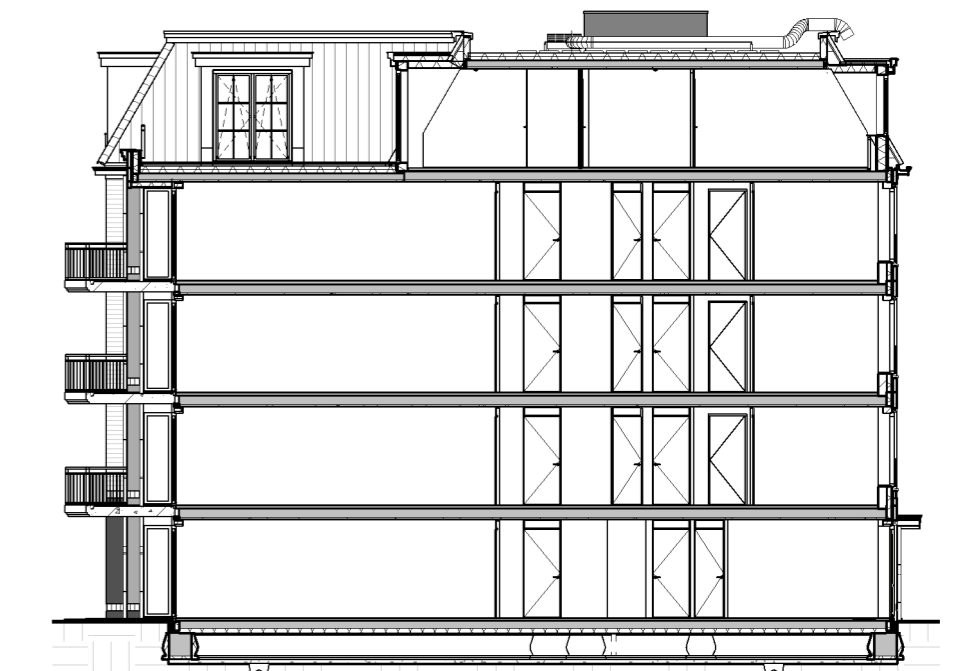
Doorsnede blok B
