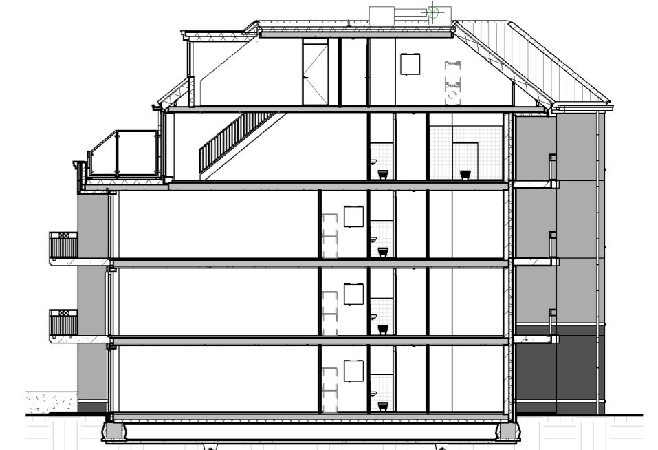
Doorsnede blok A
